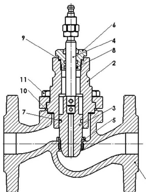
Клапан исполнение 80
